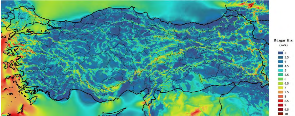
Türkiye Yıllık Ortalama Rüzgâr Hızı Dağılımı (100 Metre)
